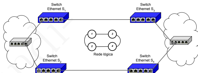
Figura 15.5: Rede com uma configuração necessária para efeitos de tolerância a falhas mas que introduz ciclos.
