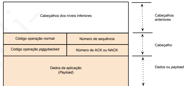
Figura 6.21: Formato das mensagens usadas pelos protocolos em conexões bidireccionais com informação piggybacked
