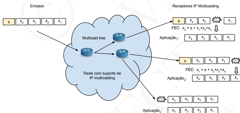
Figura 9.10: Correção de erros de omissão com multicasting usando Forward Error Correction
