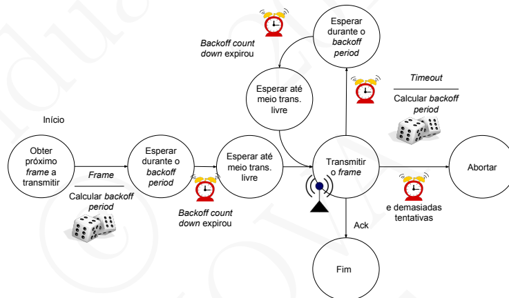
Figura 14.6: Máquina de estados usada no protocolo MAC CSMA/CA para a emissão de cada frame
