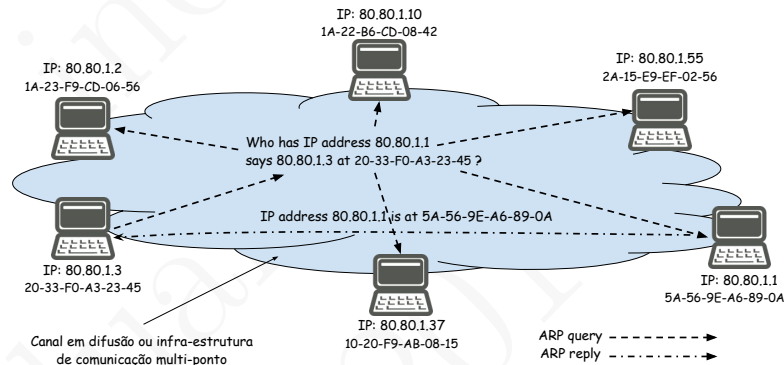
Figura 17.16: Funcionamento do protocolo ARP quando o computador com endereço 80.80.1.3 pretende descobrir o endereço MAC do computador com o endereço IP 80.80.1.1
