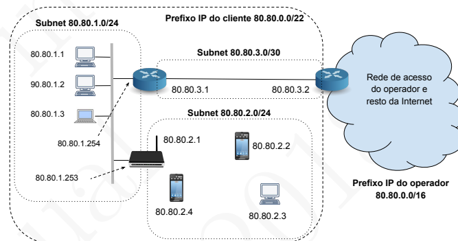
Figura 17.9: Plano de endereçamento de uma rede IP de um cliente ligado a um operador Internet
