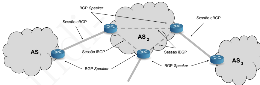
Figura 18.10: Sessões BGP estabelecidas pelos BGP speakers dentro do AS (sessões iBGP a tracejado) e os dos ASs vizinhos (sessões eBGP a traço grosso).
