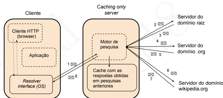
Figura 1.17: Pesquisa do endereço IP de www.wikipedia.org através de um caching only server - a numeração das mensagens segue a ordem de execução do protocolo
