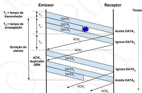
Figura 6.15: Ilustração da optimização possível na sequência de um ACK duplicado
