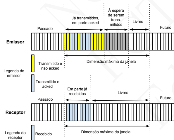
Figura 6.18: Janelas do emissor e do receptor no protocolo SR
