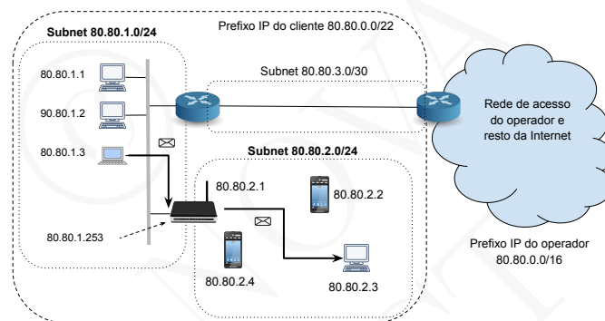
Figura 17.13: Envio de um pacote do endereço 80.80.1.3 para o endereço 80.80.2.3 através de encaminhamento indirecto.
