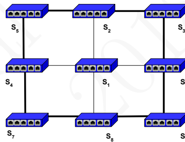
Figura 15.23: Rede de comutadores Ethernet do exercício 18.
