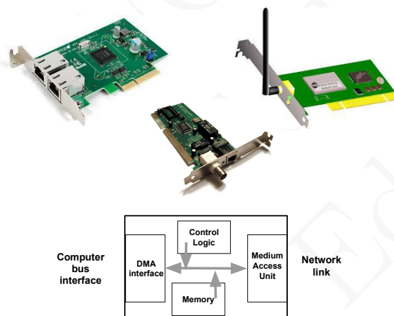
Figura 1.18: Interfaces de rede para computadores (separadas das placas mãe) e um diagrama esquemático das suas componentes
