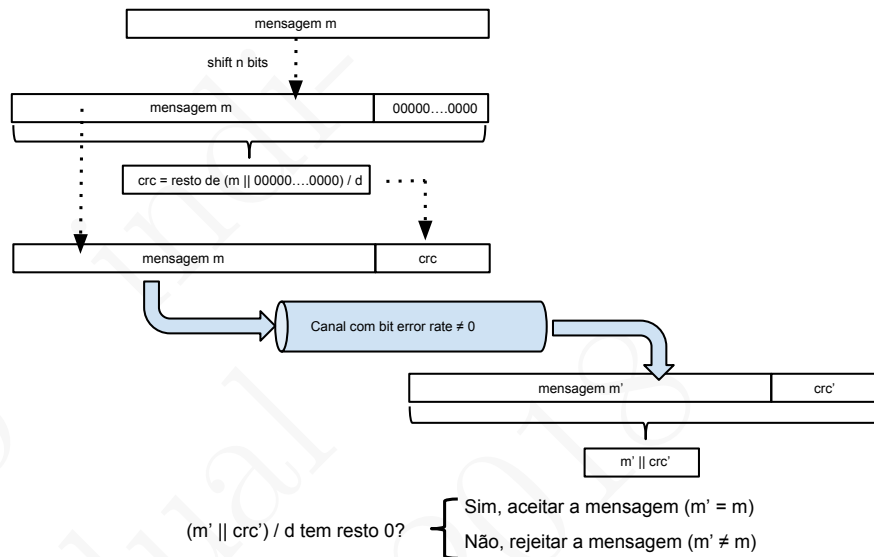
Figura 2.14: Cálculo do código de controlo de erros com o método Cyclic Redundancy Check (CRC) – '||' denota concatenação
