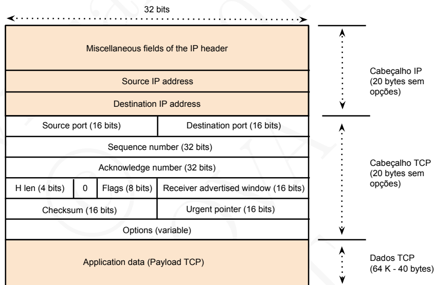
Figura 7.3: Formato de um segmento TCP
