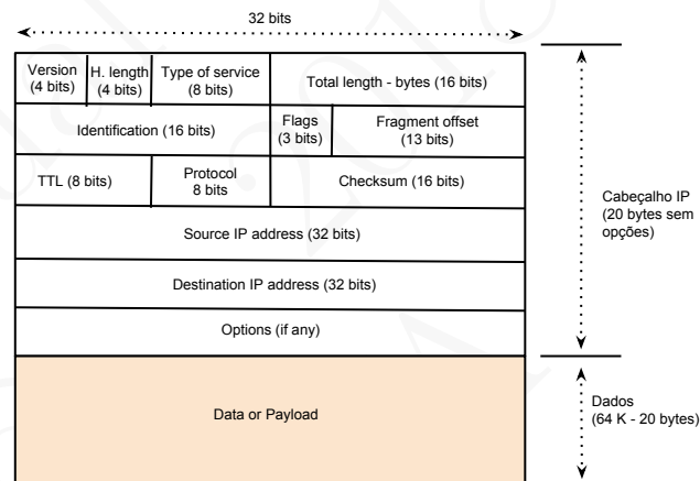
Figura 17.7: Cabeçalho de um pacote IP na versão 4
