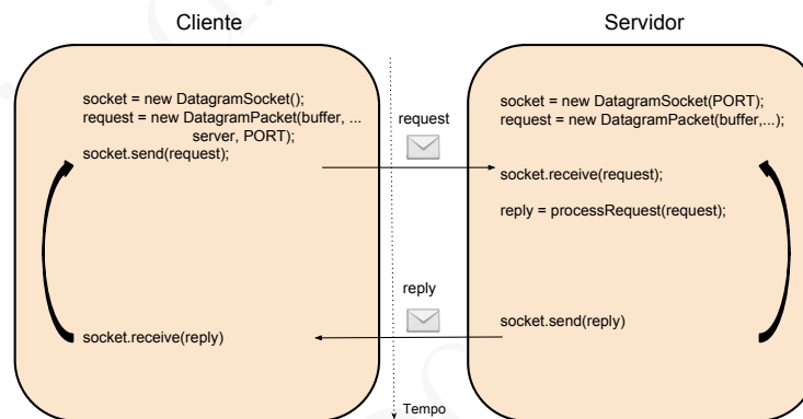
Figura 5.4: Cliente e servidor em comunicação usando sockets UDP em Java
