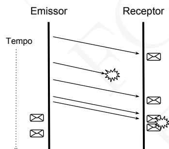
Figura 6.1: Diagrama temporal da transmissão de pacotes com informação do emissor para o receptor, com ilustração da perda de um pacote e da emissão de outro demasiado cedo
