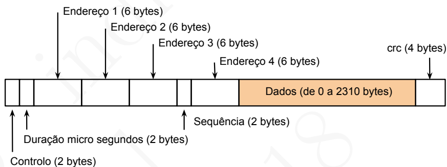
Figura 14.21: Formato dos frames IEEE 802.11
