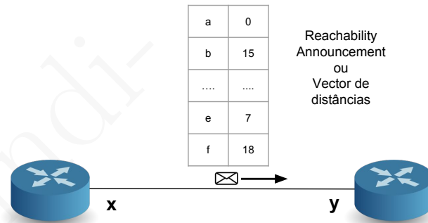
Figura 16.12: O comutador x passa a um seu vizinho y o conjunto de destinos que conhece e a que distância os consegue alcançar, através de um vector de distâncias ou reachability announcement .
