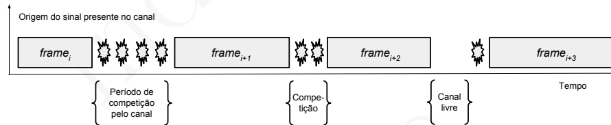
Figura 14.8: Evolução no tempo da utilização de um canal de difusão partilhado pelo protocolo CSMA/CD
