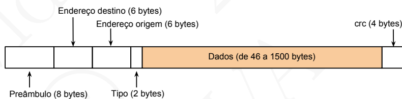
Figura 2.15: Estrutura do frame Ethernet na norma IEEE 802.3
