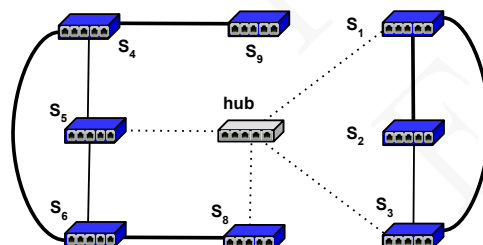
Figura 15.24: Rede de comutadores Ethernet do exercício 19.
