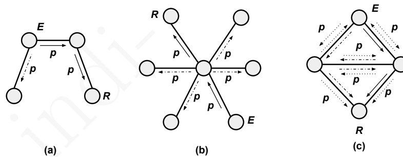
Figura 15.1: Encaminhamento por inundação do pacote p do emissor E para o receptor R . As setas correspondem a cópias do pacote: as a negro são as necessárias; as a ponto e traço são inúteis; e as a ponteadas são algumas das cópias duplicadas.
