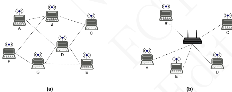
Figura 14.17: Modo ad hoc (a) e modo infra-estrutura (b). Neste último um ponto de acesso serve como intermediário das comunicações entre as diversas estações
