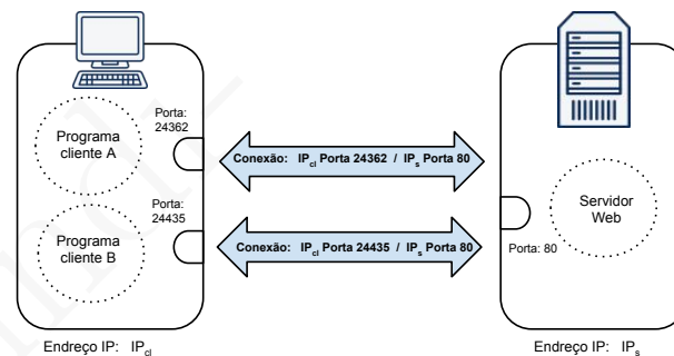
Figura 7.2: Endereços IP e portas envolvidos em duas conexões TCP entre um mesmo computador cliente e o mesmo servidor HTTP
