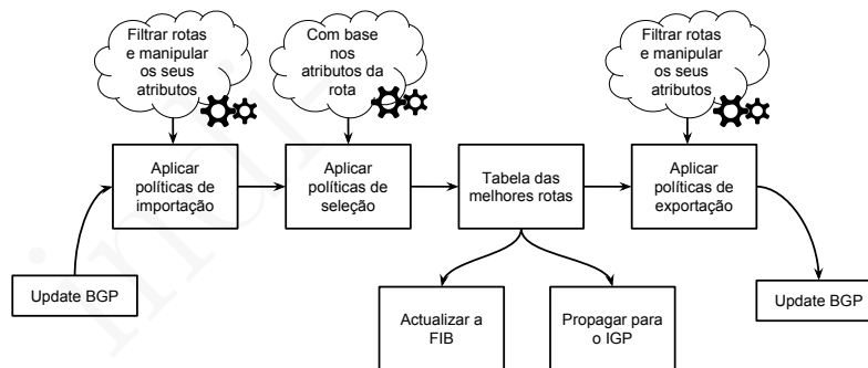
Figura 18.14: Passos seguidos desde que um BGP update é recebido até que o mesmo se repercute na FIB do router, é propagado aos outros routers através do IGP e dá origem a outro(s) update(s) enviados para outros ASs.
