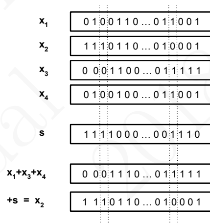
Figura 9.8: Cálculo do pacote sumário e sua utilização para calcular o valor de um pacote em falta
