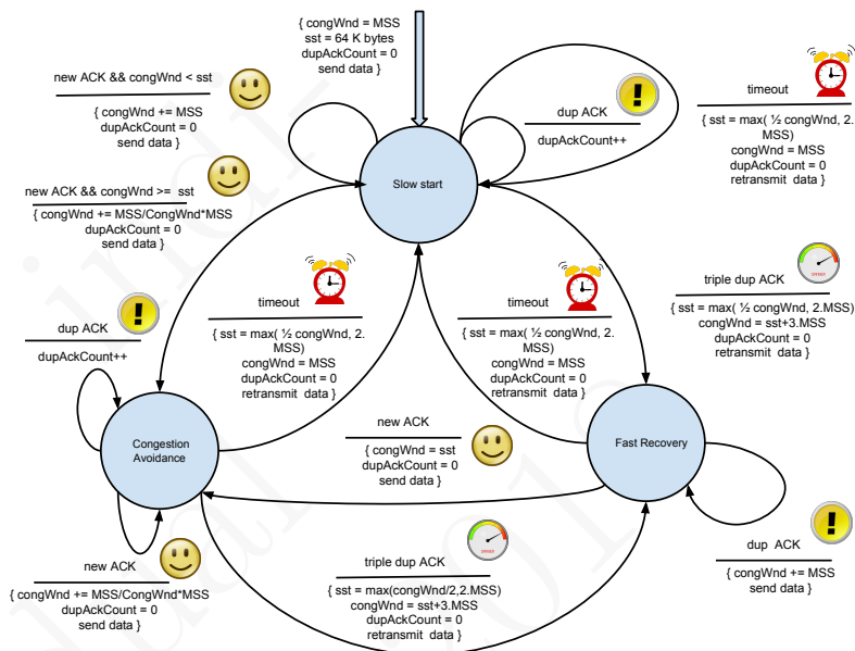
Figura 8.19: Descrição do algoritmo de controlo da saturação TCP Reno
