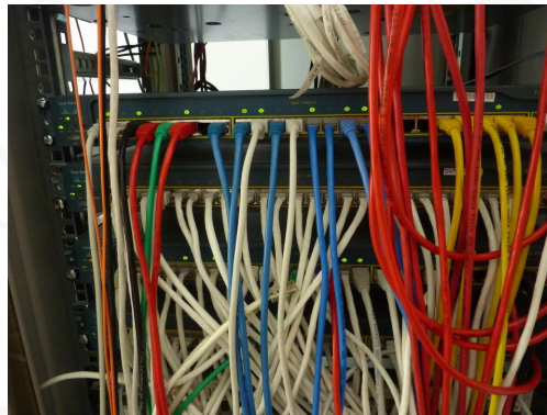
Figura 2.8: Interligação de muitos computadores através de vários comutadores pondo em evidência a complexidade da gestão dos cabos UTP nesse cenário
