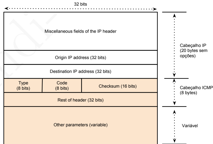
Figura 17.18: Formato das mensagens do protocolo ICMPv4
