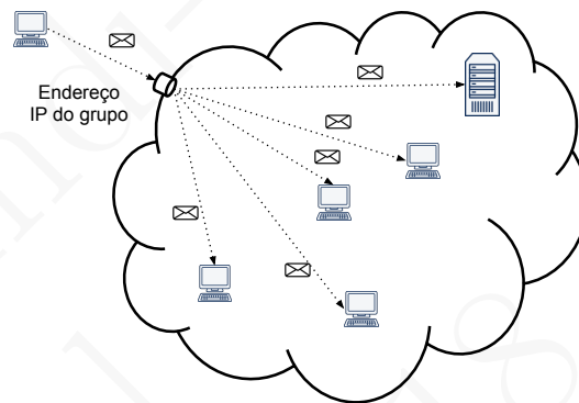
Figura 5.5: Difusão através de IP Multicasting de um datagrama para um grupo de computadores
