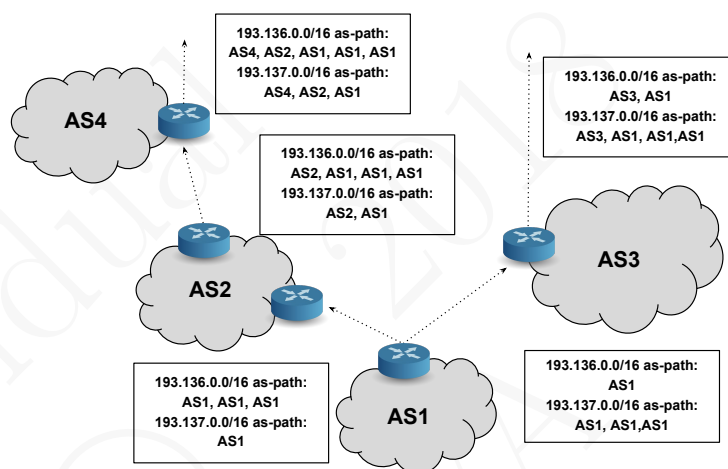
Figura 18.17: Utilização de repeated AS prepending para influenciar a distribuição do tráfego de entrada num AS multi-homed .
