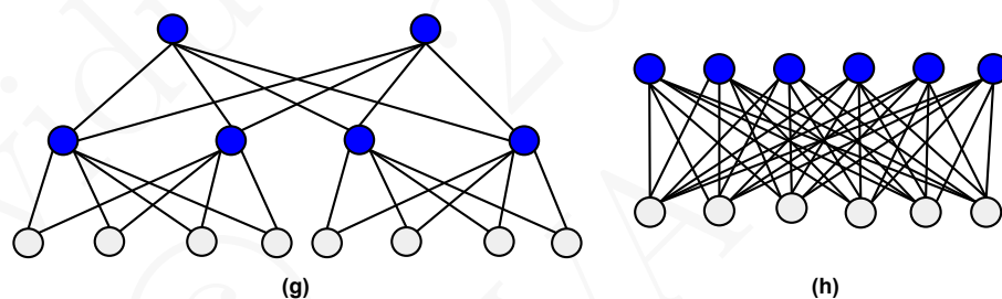
Figura 4.7: Redes (g) Hierárquica duplicada, também conhecida por Fat tree , e (h) Clos network
