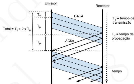
Figura 6.11: Aumento da velocidade de transferência extremo a extremo pelo aumento do número de pacotes in-flight
