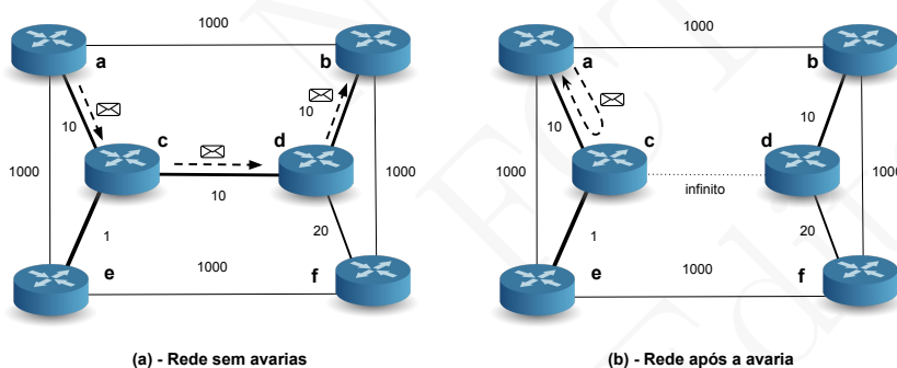
Figura 16.10: Antes da avaria do canal entre os comutadores c e d, parte (a), os pacotes que vão de a para b seguem via o caminho a, c, d, b por este ser o mais curto. Depois da avaria, parte (b), o comutador c acha que o melhor caminho é via a, b mas o comutador a ainda não actualizou a sua FIB e os pacotes entram em ciclo.
