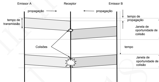
Figura 14.4: Com a versão Slotted ALOHA a oportunidade de colisões é menor
