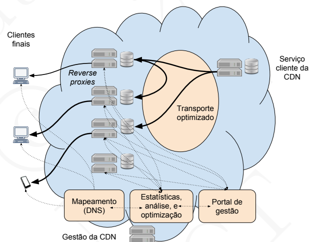
Figura 13.7: Estrutura interna de uma CDN com os proxies inversos em diferentes regiões geográficas e os servidores centrais de controlo e gestão. As linhas a negrito representam os fluxos de dados. As linhas a tracejado os fluxos de controlo. Adaptado de [Nygren et al., 2010].
