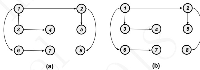
Figura 15.3: A difusão não introduz duplicados numa rede estruturada em árvore. No caso (a) o emissor é o nó 3 e no caso (b) é o nó 1.
