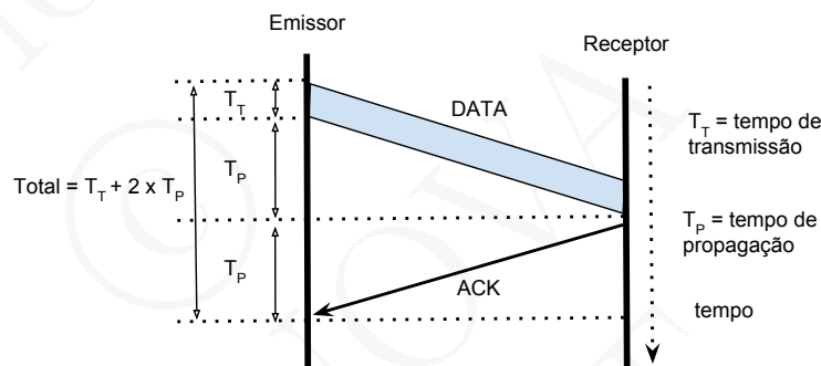
Figura 6.9: Determinação do desempenho do protocolo stop & wait
