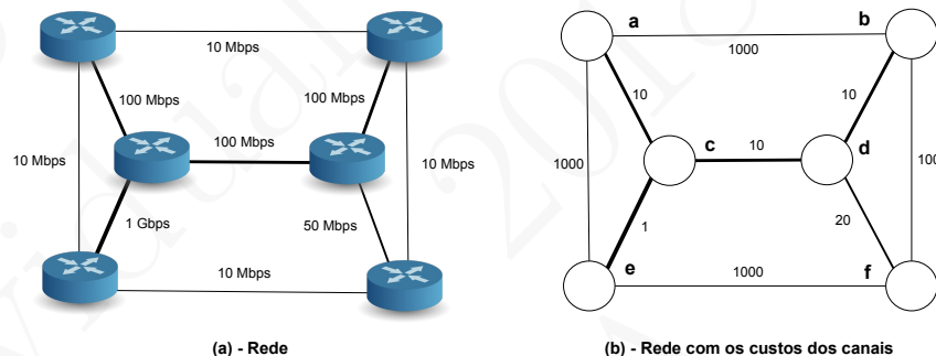
Figura 16.6: Rede e informações necessárias para preencher a LSDB da mesma
