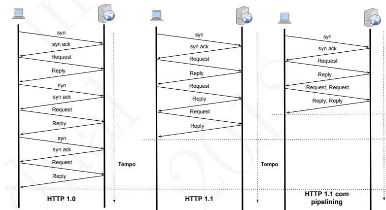
Figura 12.6: Tempo para obter uma página Web e dois objectos nela referenciados com diferentes versões do protocolo HTTP. O diagrama ignora o ganho suplementar devido a só existir, potencialmente, uma única fase slow start da conexão e considera, por hipótese, que cada pedido e resposta são executados num único RTT.
