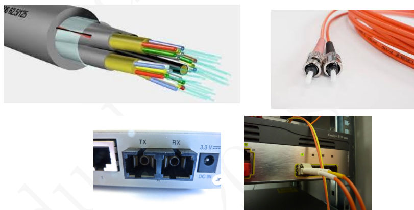
Figura 2.7: Cabo com várias fibras ópticas, “chicote” de fibra óptica e fichas de ligação a interfaces. Cada canal full-duplex usa um par de fibras (TX - Transmitir, RX - Receber)
