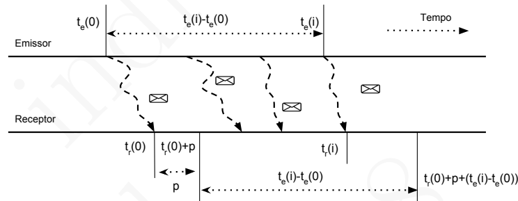
Figura 3.15: Utilização de marcas temporais, de um playback buffer e de um playout delay ( P ) para compensar o jitter
