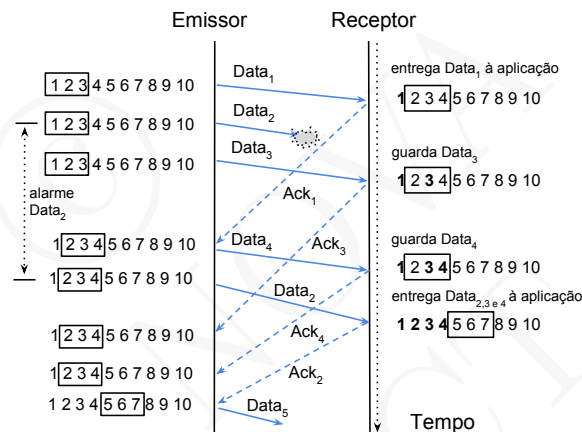
Figura 6.19: O protocolo SR em acção, com recuperação mais rápida do erro e sem retransmissão de pacotes já recebidos pelo receptor
