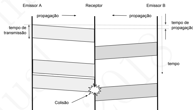
Figura 14.2: Emissores ligados ao mesmo meio de comunicação - se as emissões tiverem lugar em momentos diferentes, não há colisão; senão os frames colidem e o receptor recebe-os com erros
