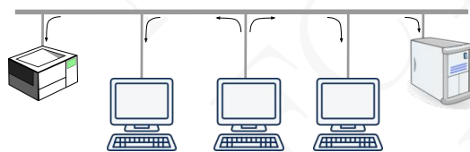
Figura 14.11: Um conjunto de computadores interligados a 10 Mbps por uma rede Ethernet 802.3 baseada num cabo coaxial partilhado entre os diferentes computadores
