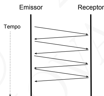
Figura 6.2: Diagrama temporal da transmissão de pacotes com informação do emissor para o receptor e de pacotes de controlo no sentido contrário
