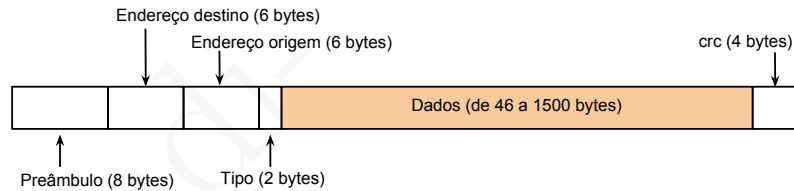
Figura 14.9: Formato dos frames Ethernet
