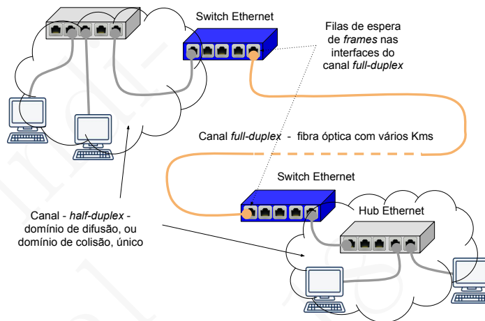
Figura 14.13: Coexistência na mesma rede Ethernet 802.3 de hubs e switches Ethernet e de canais half e full-duplex
