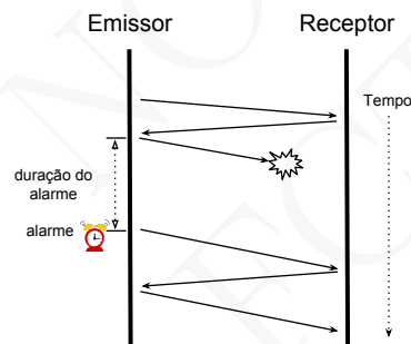
Figura 6.4: Utilização de um temporizador para desbloquear uma situação de bloqueamento por perda de pacotes
