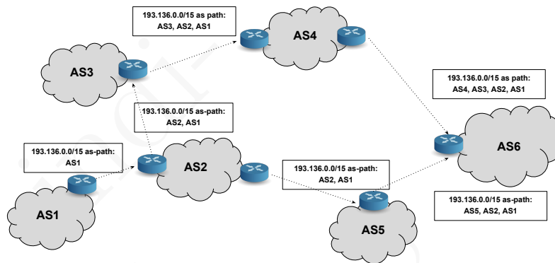
Figura 18.13: Propagação dos AS paths através dos ASs e recepção por um AS de mais do que uma rota para o mesmo prefixo.
