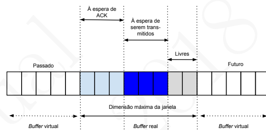
Figura 6.12: Janela do emissor nos protocolos de janela deslizante
