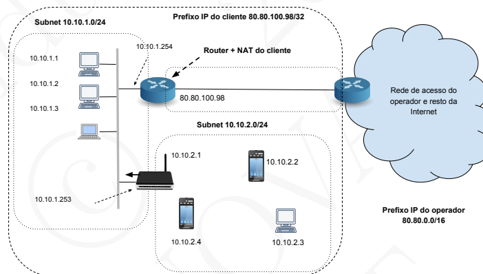
Figura 17.19: Rede de um cliente baseada em endereçamento privado
