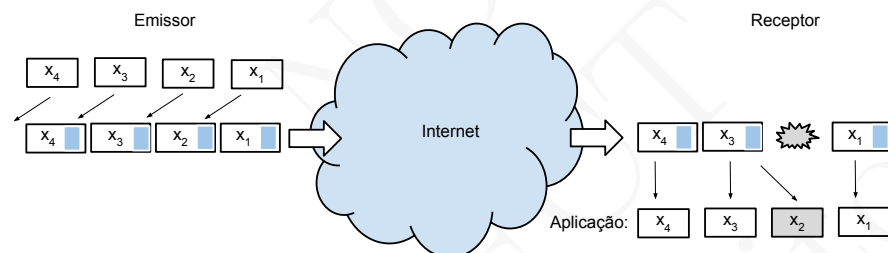
Figura 9.13: Forward Error Correction com base num codec de resolução inferior
