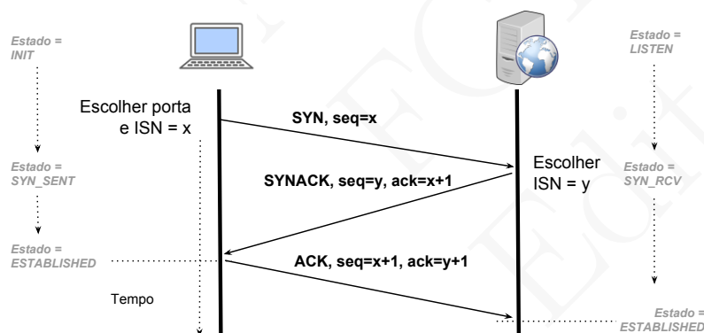
Figura 7.11: Abertura de uma conexão TCP. À esquerda a parte que solicita a abertura, à direita a que aceita a conexão
