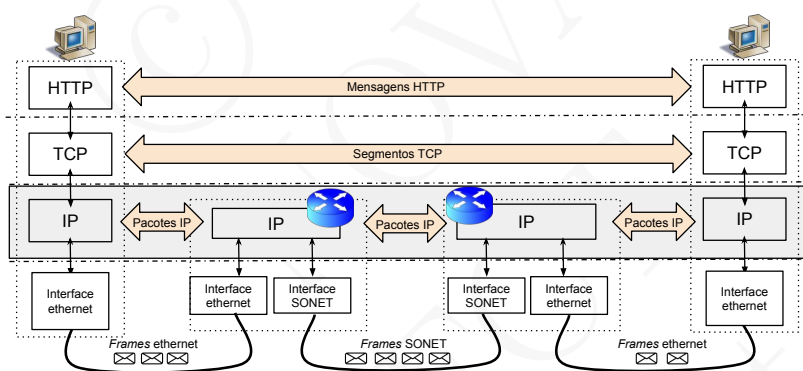
Figura 13.15: O nível rede (a sombreado) utiliza canais de dados e comutadores de pacotes para providenciar os seus serviços aos níveis superiores
