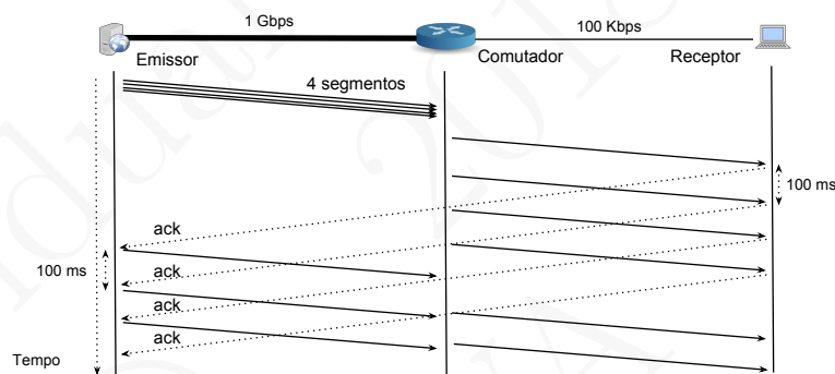
Figura 8.12: O débito do canal gargalo impõe o ritmo de chegada de ACKs e também o ritmo de envio de segmentos pelo emissor
