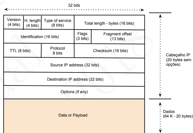
Figura 1.3: Pacote IP - campos do cabeçalho do pacote e parte de dados
