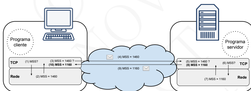
Figura 7.4: Na abertura da conexão, as partes acordam o valor do MSS (os números das legendas denotam a ordem das operações)
