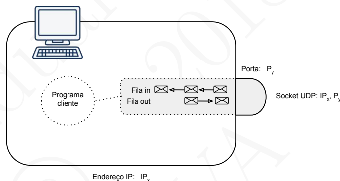
Figura 5.3: Filas de espera associadas a um socket UDP
