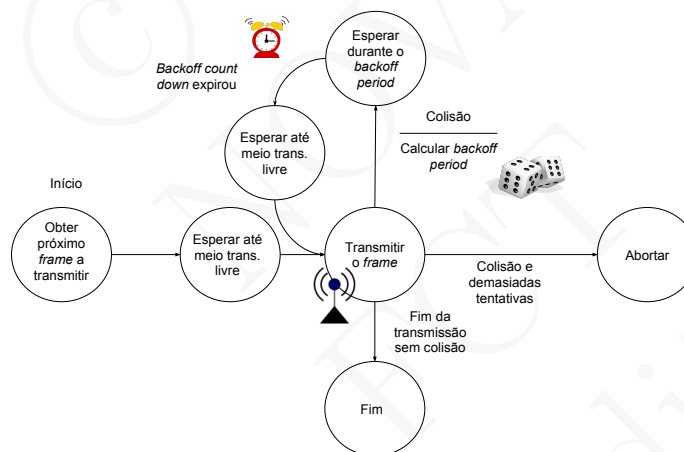
Figura 14.7: Máquina de estados usada no protocolo MAC CSMA/CD para a emissão de cada frame
