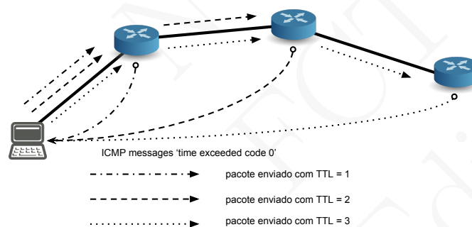
Figura 3.13: Execução do programa traceroute
