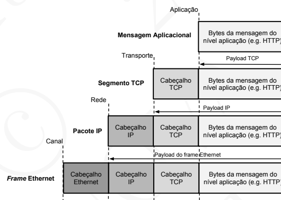
Figura 4.13: Cabeçalhos e encapsulamento nos diferentes níveis
