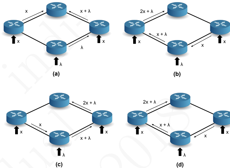
Figura 16.11: Considerar a intensidade do tráfego ou a dimensão das filas de espera de forma significativa na métrica do custo de um canal pode conduzir a instabilidade no encaminhamento.
