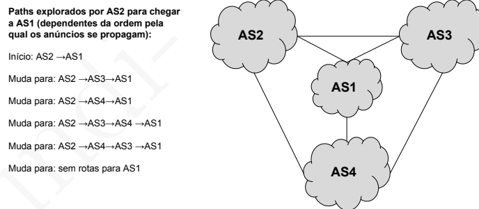
Figura 18.18: Instabilidade introduzida pela path exploration quando o AS1 deixou de estar acessível. Evolução dos caminhos usados por AS2 para chegar a AS1 até concluir que este deixou de estar acessível. Uma evolução semelhante passa-se também com o AS3 e o AS4.
