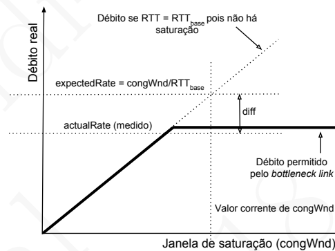
Figura 8.25: TCP Vegas: expectedRate e actualRate de uma conexão
