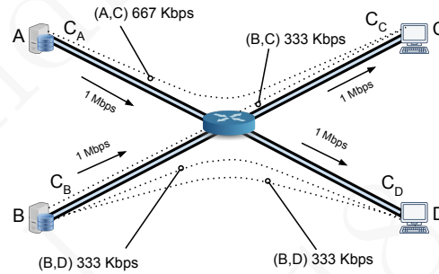
Figura 8.10: Determinação do débito máximo dos fluxos (A,C), (B,C) e 2 \times (B,D) numa rede em estrela
