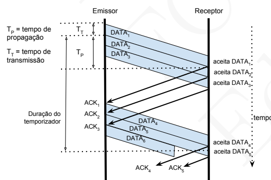
Figura 6.13: O protocolo GBN evoluindo sem erros
