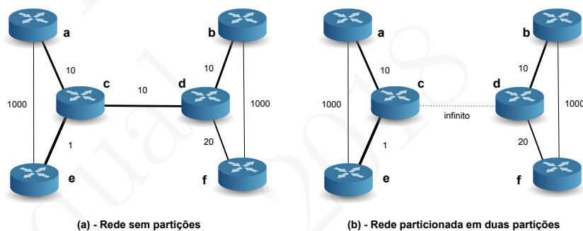
Figura 16.9: Rede completa com todos os canais operacionais (a). Na sequência da avaria do canal entre os comutadores c e d, a rede fica particionada em duas incomunicáveis entre si (b).
