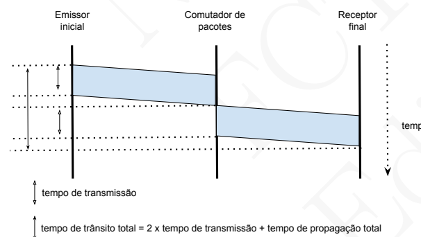
Figura 3.9: Atraso introduzido devido ao tempo de transmissão
