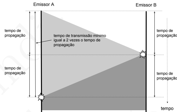
Figura 14.10: O emissor A começa a emitir, mas mesmo antes que o seu sinal chegue a B, este, julgando o meio livre, começa a emitir. B detecta imediatamente a colisão, mas A só detecta a colisão quando o sinal de B se propagar até ele, i.e. , ao fim de 2 \times T_p .
