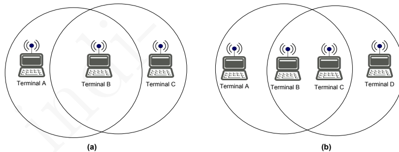
Figura 14.16: Em (a) os terminais A e C estão suficientemente afastados para não receberem os respectivos sinais com intensidade suficiente para detectarem a colisão que ocorre em B. Em (b) apesar de B e C estarem expostos aos respectivos sinais, B poderia emitir para A ao mesmo tempo que C emitiria para D.
