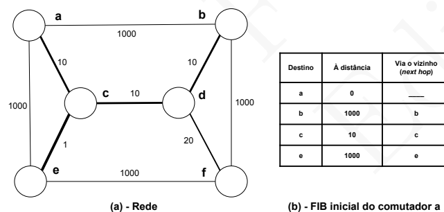
Figura 16.13: Rede usada no exemplo e FIB inicial do comutador a
