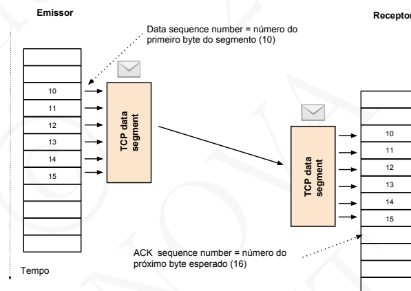
Figura 7.6: Números de sequência e de ACK dos segmentos
