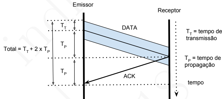
Figura 6.20: Progresso de um protocolo de janela deslizante sem erros e com N = 2
