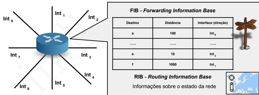
Figura 16.5: Computador de pacotes e as duas bases de informação: FIB - Forwarding Information Base e RIB - Routing Information Base
