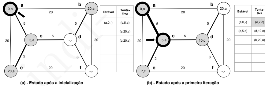
Figura 16.2: Estado do grafo após a inicialização do algoritmo (a) e o mesmo estado após a primeira iteração (b). À direita de cada grafo figura a visão do encaminhamento pelo nó a .
