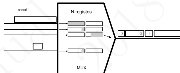
Figura 3.6: Multiplexagem estatística
