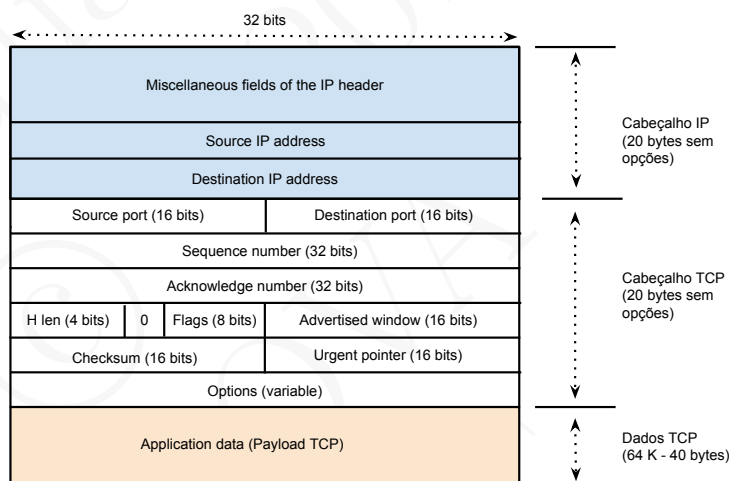
Figura 1.8: Segmento TCP e campos do seu cabeçalho
