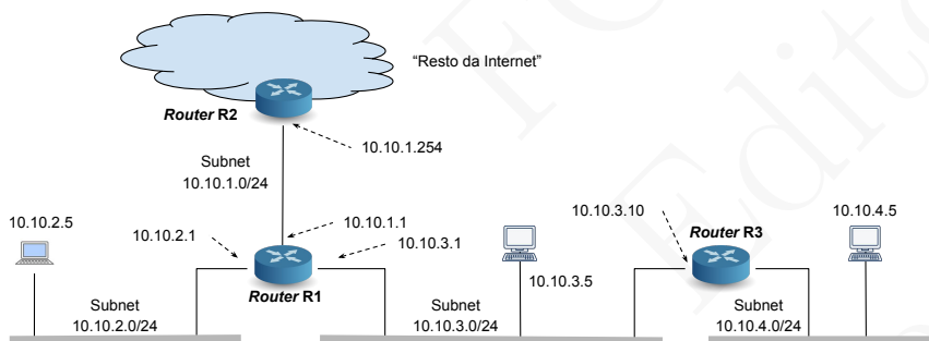
Figura 17.24: Rede ligada à Internet através de um ISP
