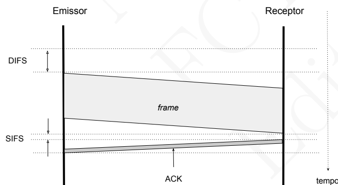
Figura 14.19: Funcionamento do MAC IEEE 802.11 e os respectivos compassos de espera DIFS e SIFS
