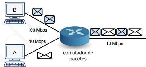
Figura 3.11: Os computadores A e B estão ligados via o comutador de pacotes em cuja interface de saída se forma uma fila de espera
