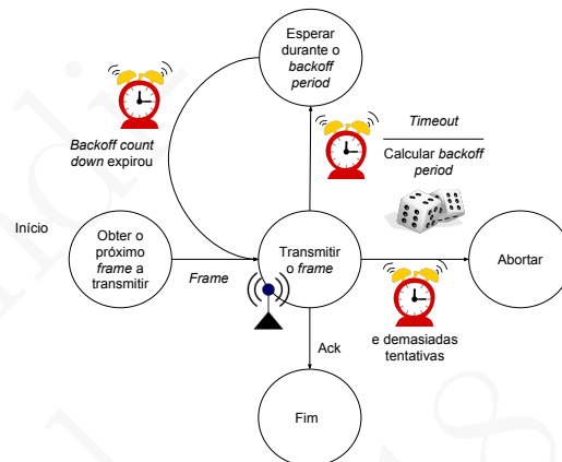
Figura 14.3: Máquina de estados usada no protocolo MAC ALOHA para a emissão de cada frame
