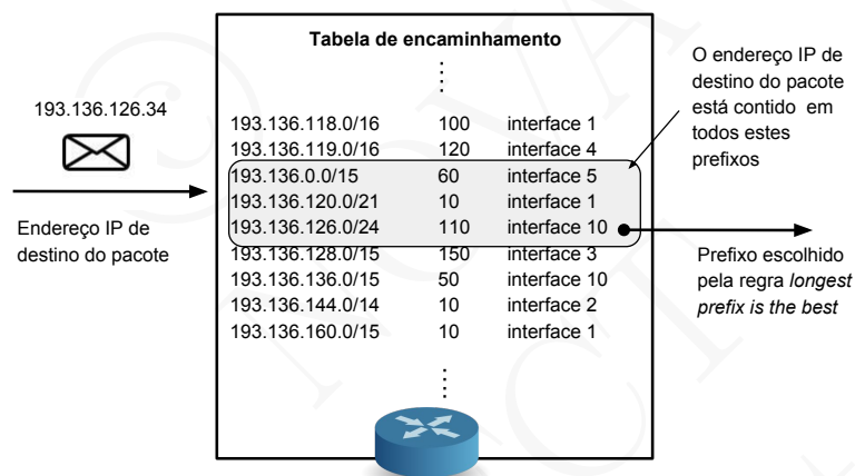
Figura 17.5: Tabela de encaminhamento IP e a regra longest prefix is the best
