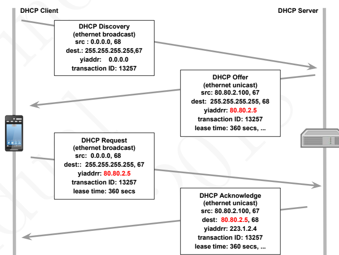
Figura 17.17: Funcionamento do protocolo DHCP
