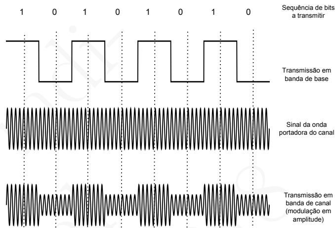
Figura 2.11: Codificação de uma sequência alternada de 0s e 1s em banda de base e em banda de canal com modulação em amplitude da portadora
