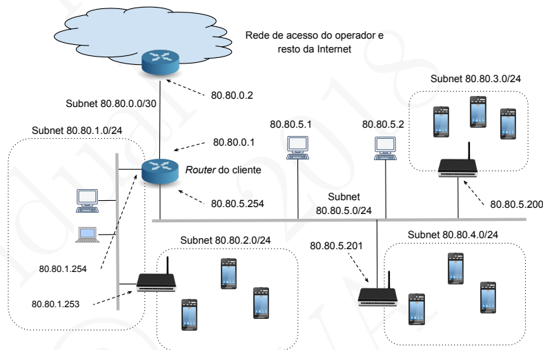
Figura 17.23: Rede de um cliente ligada à Internet através de um ISP
