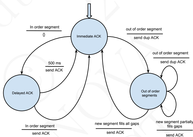
Figura 8.16: Funcionamento do receptor TCP
