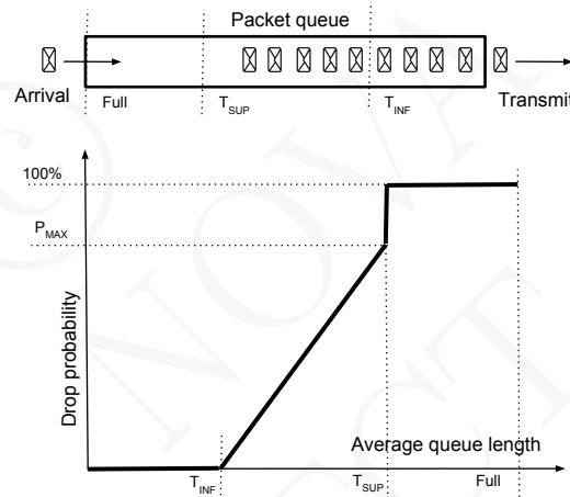
Figura 8.22: Função probabilidade de supressão de pacotes com RED
