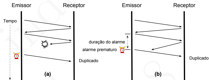
Figura 6.5: A perda de um pacote de controlo (a) ou um alarme prematuro (b) conduzem à recepção de um pacote em duplicado
