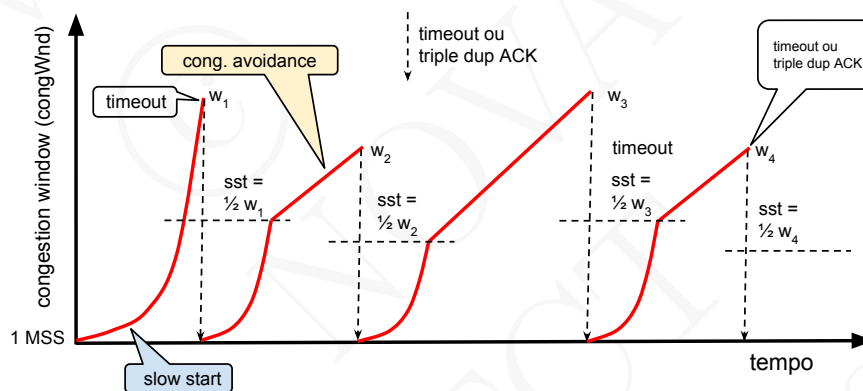
Figura 8.17: Evolução do valor do limite congWnd ao longo de uma conexão TCP na versão TCP Tahoe
