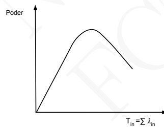
Figura 8.9: Poder da rede em função de T_{in}
