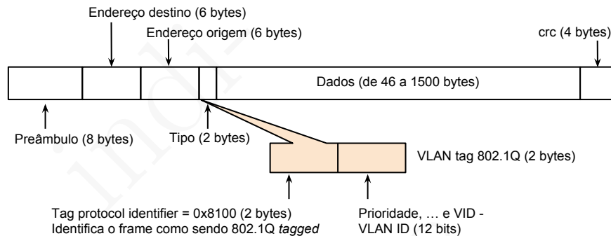
Figura 15.13: Formato dos frames Ethernet que incluem o cabe alho IEEE 802.1Q. O valor que indica a presen a deste foi escolhido de tal forma que permite distinguir um frame 802.1Q de um convencional pois   diferente de todos os valores legais do campo Tipo.
