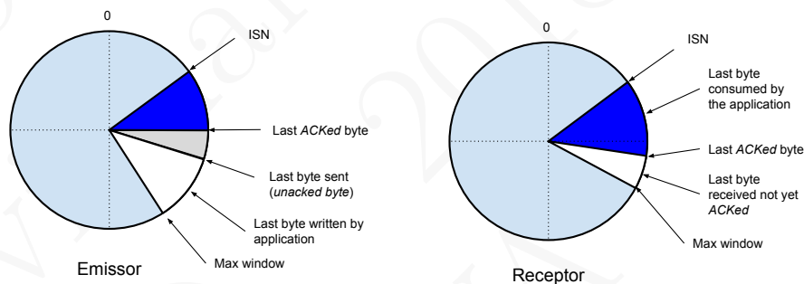
Figura 7.10: Visão da utilização dos números de sequência por cada um dos lados da conexão TCP como um relógio
