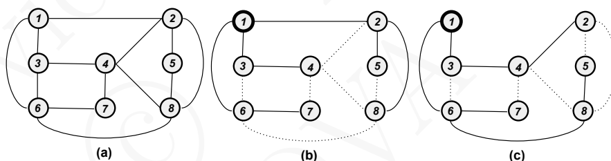
Figura 15.6: Papel do protocolo STP: (a) rede completa, (b) uma sub-rede calculada pelo STP, (c) outra sub-rede calculada pelo STP após a avaria do canal que liga os nós 1 e 2.
