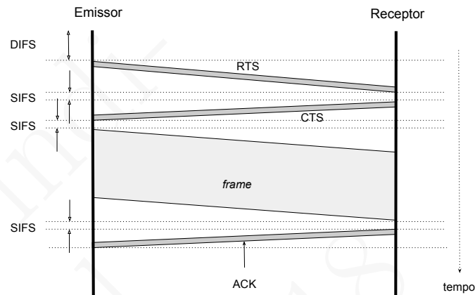
Figura 14.20: Funcionamento do MAC IEEE 802.11 utilizando o mecanismo RTS / CTS
