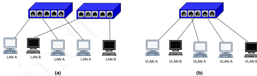
Figura 15.11: Duas redes distintas fisicamente (a) e uma implementação equivalente através de um único switch e duas VLANs distintas (b).
