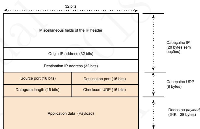
Figura 1.14: Formato de um datagrama UDP
