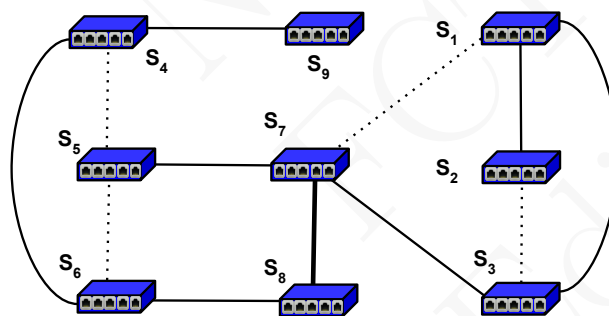
Figura 15.22: Rede de comutadores Ethernet do exercício 17.
