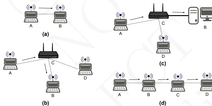
Figura 14.22: Vários cenários de comunicação entre terminais que ilustram a necessidade de usar mais do que dois endereços no cabeçalho dos frames IEEE 802.11 (situações (b), (c) e (d))
