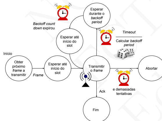
Figura 14.5: Máquina de estados usada no protocolo MAC Slotted ALOHA para a emissão de cada frame
