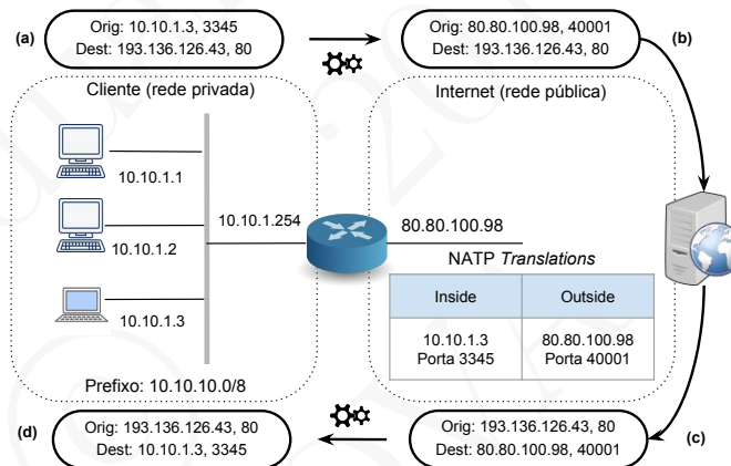
Figura 17.20: Tradução de endereços com base em portas (NATP)
