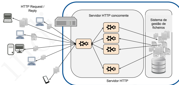
Figura 12.7: Servidor HTTP processando múltiplas conexões HTTP em paralelo através de diversos threads de execução
