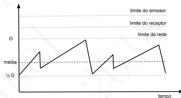
Figura 8.24: Débito de uma conexão TCP idealizada
