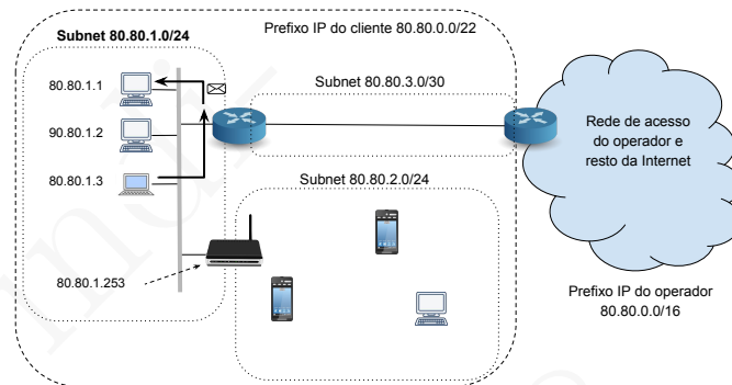
Figura 17.11: Envio de um pacote do computador com o endereço 80.80.1.3 para o com o endereço 80.80.1.1 através de encaminhamento directo.
