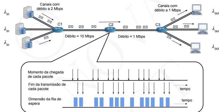
Figura 8.3: Filas de espera no interior da rede com T_{out} = T_{in}
