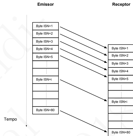
Figura 7.5: Números de sequência dos bytes no TCP
