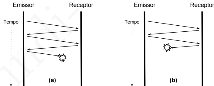
Figura 6.3: Bloqueio da transferência por (a) perda de um pacote com informação ou por (b) perda de um pacote de controlo
