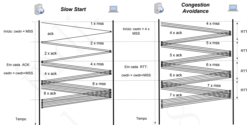
Figura 8.15: Subida da janela de emissão durante a fase slow start e durante a fase congestion avoidance do TCP
