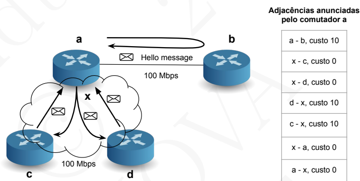
Figura 16.8: Entre os comutadores directamente ligados a um canal multi-ponto, um é eleito designated router e passa a ser responsável por um pseudo comutador, com o objectivo de evitar a explosão do número de canais ponto-a-ponto da rede.
