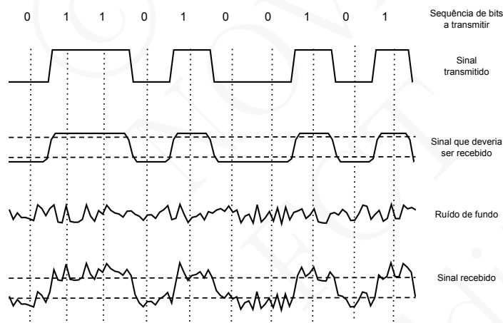
Figura 2.12: O sinal digital original emitido é degradado, quer pela propagação do mesmo pelo canal, quer pela presença de ruído no canal
