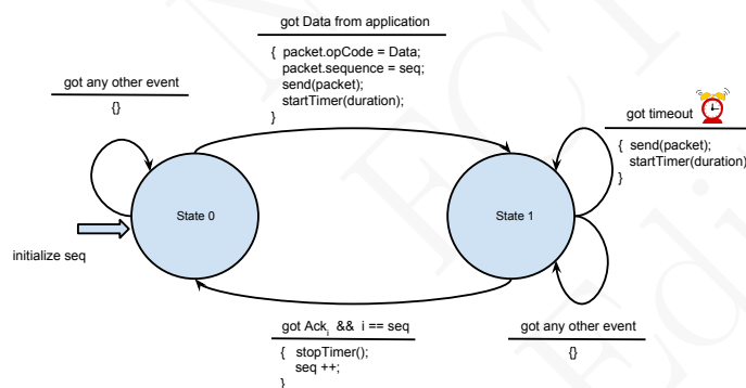
Figura 6.23: Máquina de estados do emissor stop & wait
