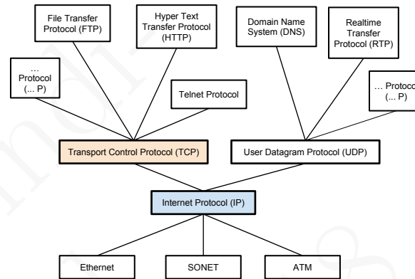
Figura 4.12: Exemplos de protocolos dos diferentes níveis da pilha de protocolos TCP/IP
