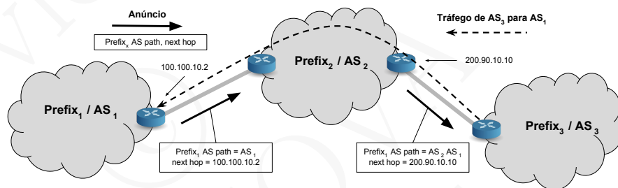
Figura 18.4: Forma e propagação dos anúncios BGP e como os mesmos atraem o tráfego dirigido ao prefixo anunciado.
