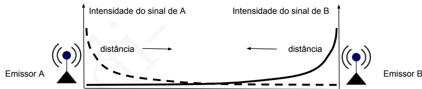
Figura 14.14: Os terminais A e B estão suficientemente afastados para não receberem os respectivos sinais com intensidade suficiente para detectarem a colisão
