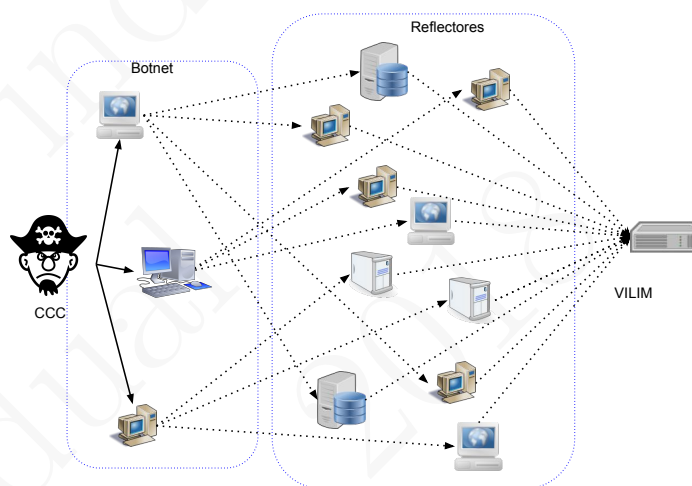
Figura 4.4: Ataque de negação de serviço distribuído por reflexão: CCC, através da sua botnet , ataca o computador VILIM
