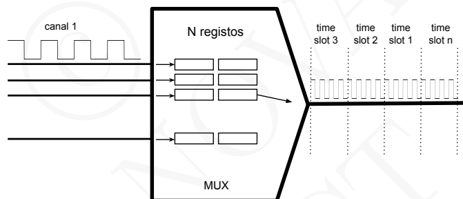
Figura 3.4: Multiplexagem por tempo
