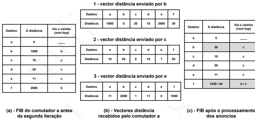
Figura 16.16: (a) FIB do computador a antes da segunda iteração. (b) vectores distância recebidos dos vizinhos de a. (c) FIB do computador a após a segunda iteração.
