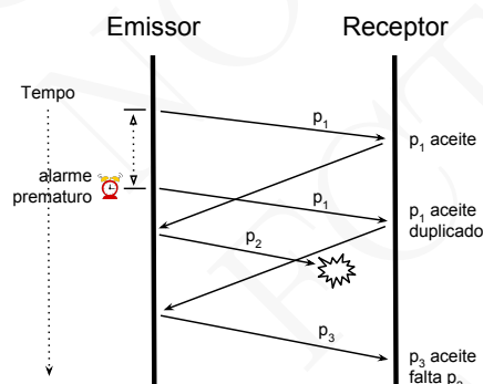
Figura 6.6: Duplicado de um pacote por o alarme ocorrer demasiado cedo, seguido da perda não detectada de um pacote
