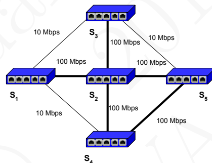
Figura 15.17: Rede de comutadores Ethernet do exercício 12.
