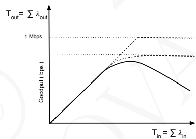
Figura 8.7: Goodput com filas de espera finitas, retransmissão prematura de pacotes atrasados e supressão de pacotes que consumiram recursos no bottleneck link antes de serem suprimidos
