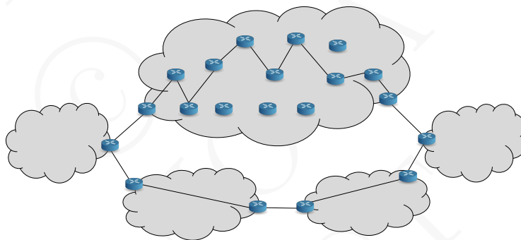
Figura 18.15: Comparar rotas pelo número de ASs pode revelar-se enganador.
