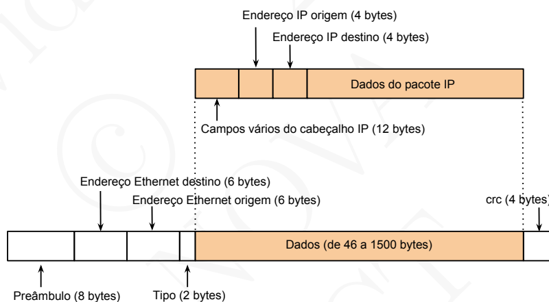
Figura 2.16: Encapsulamento de um pacote IP num frame Ethernet
