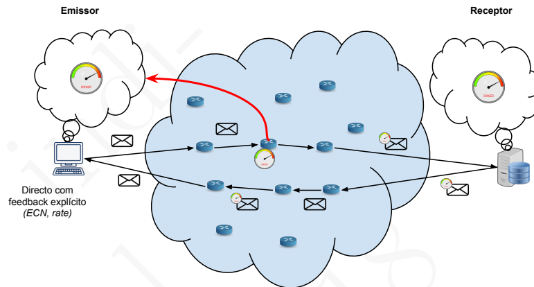
Figura 8.20: Encaminhamento de feedback explícito encavalitado no tráfego enviado no sentido contrário
