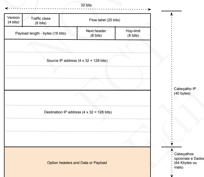
Figura 17.8: Cabeçalho de um pacote IP na versão 6
