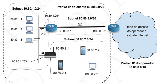
Figura 17.14: Envio de um pacote do endereço 80.80.1.3 para o endereço 193.136.126.43 através de encaminhamento por default .
