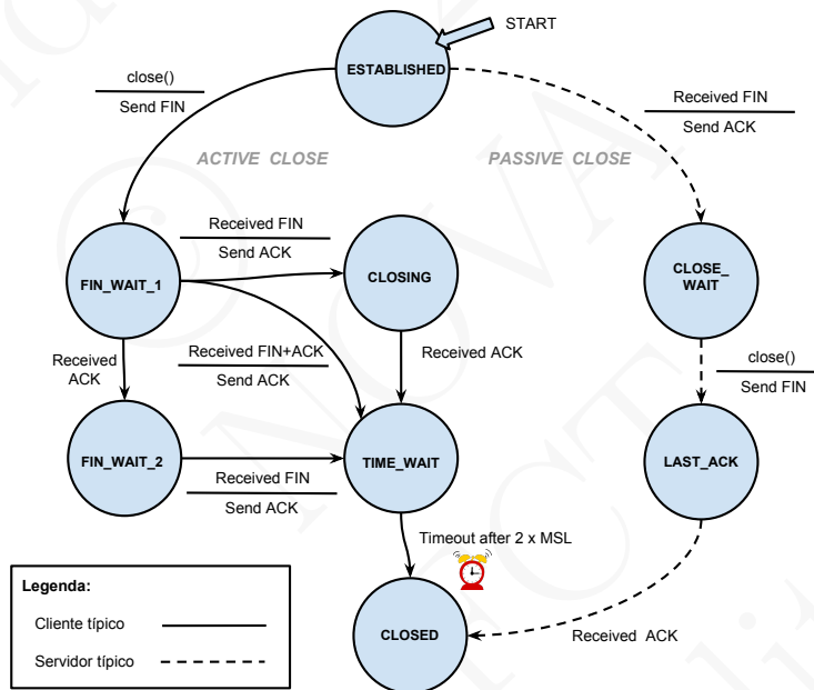
Figura 7.14: Máquina de estados correspondente ao fecho de uma conexão TCP
