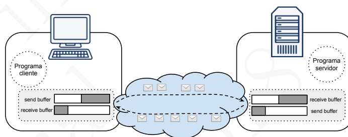
Figura 7.1: Os buffers envolvidos numa conexão TCP
