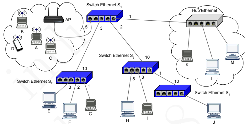
Figura 15.4: Rede com diferentes tipos de comutadores e de canais com encaminhamento por inundação e aprendizagem pelo caminho inverso.
