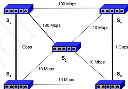
Figura 15.16: Rede de comutadores Ethernet do exercício 11.
