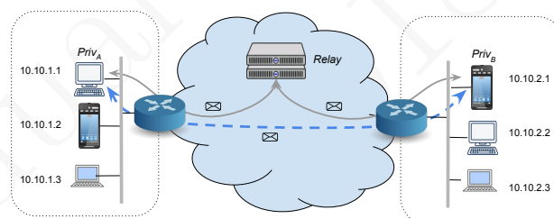
Figura 17.22: Comunicação entre dois dispositivos IP em redes privadas usando um servidor de relaying . A cheio o trajecto dos pacotes reais, a tracejado o trajecto lógico dos pacotes.
