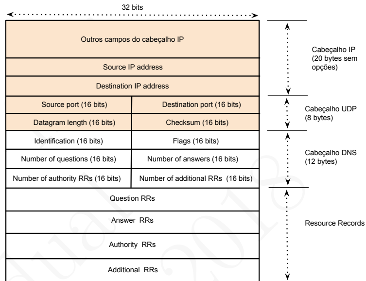
Figura 11.7: Mensagem de pedido e resposta ao DNS transportada pelo protocolo UDP
