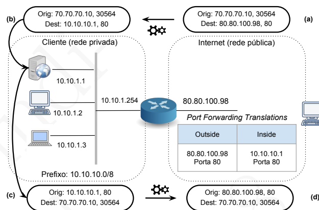
Figura 17.21: Acesso a um servidor interno com base em port forwarding
