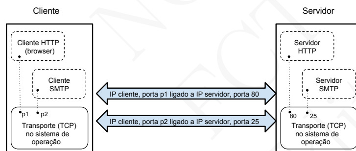
Figura 1.9: Diferentes canais TCP nos mesmos computadores distinguem-se por portas distintas
