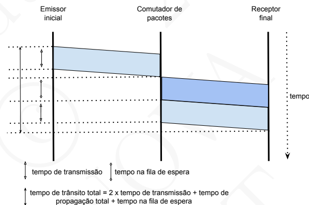
Figura 3.10: Atraso introduzido devido ao tempo de transmissão dos pacotes que já estavam na fila de espera (a mais escuro) e atraso introduzido devido ao tempo de transmissão do pacote
