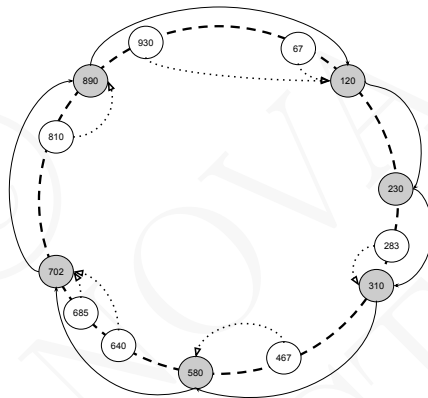
Figura 13.13: Organização lógica de um conjunto de identificadores em anel. Os nós a cinzento representam nós físicos da rede. Os restantes representam chaves de conteúdos. As setas a negro representam as ligações entre nós físicos. As setas a tracejado representam a ligação da chave k ao nó sucessor(k) , nó responsável por memorizar o valor associado a k . O domínio das chaves é de 0 a 1023.
