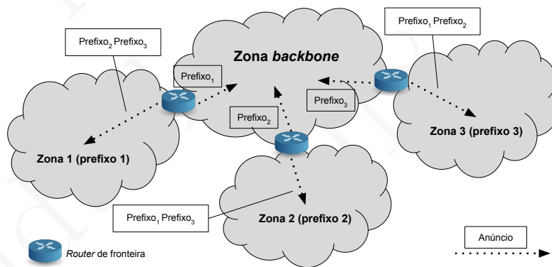
Figura 18.1: Organização de uma rede OSPF em várias zonas.
