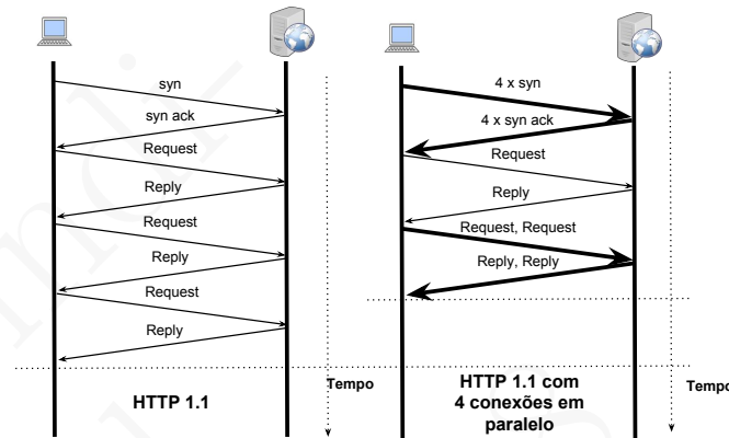
Figura 12.8: Tempo para obter uma página Web e dois objectos nela referenciados com uma conexão TCP e sem pipelining , e com 4 conexões TCP paralelas. O diagrama considera, por hipótese, que cada pedido e resposta é executado num único RTT.
