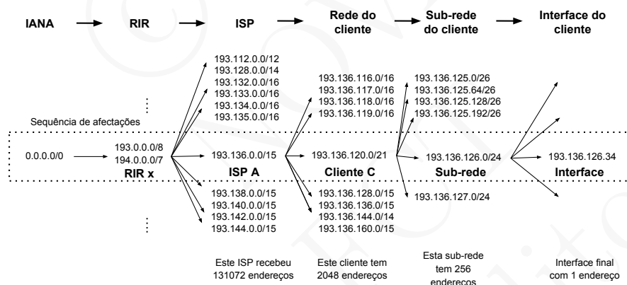
Figura 17.4: Sequência de fectações de prefixos IP: à RIR x, ao ISP A, ao cliente C etc. que permitem a afectação de um endereço a uma interface na rede do cliente C.
