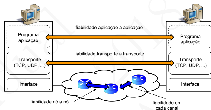
Figura 4.1: Diversas opções para garantir a fiabilidade do transporte dos dados: canal a canal, nó a nó, no protocolo de transporte, nas aplicações
