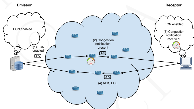
Figura 8.21: Funcionamento do mecanismo TCP ECN
