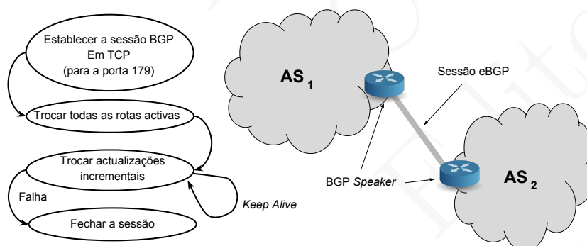
Figura 18.11: Estabelecimento das sessões BGP e fases da sessão.
