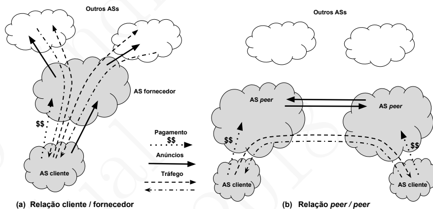
Figura 18.5: Relações entre ASs clientes e fornecedores (a) e relações entre ASs peers (b). Fluxos de anúncios dos prefixos, do tráfego e do dinheiro.
