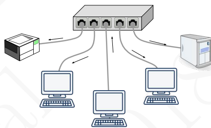
Figura 14.12: Um conjunto de computadores interligados por uma rede Ethernet 802.3 baseada em cabos UTP e um repetidor de sinal ( hub Ethernet)
