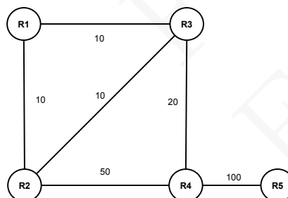
Figura 16.19: Rede do exercício 11
