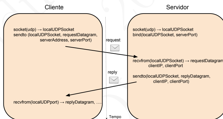
Figura 1.19: Comunicação com sockets UDP
