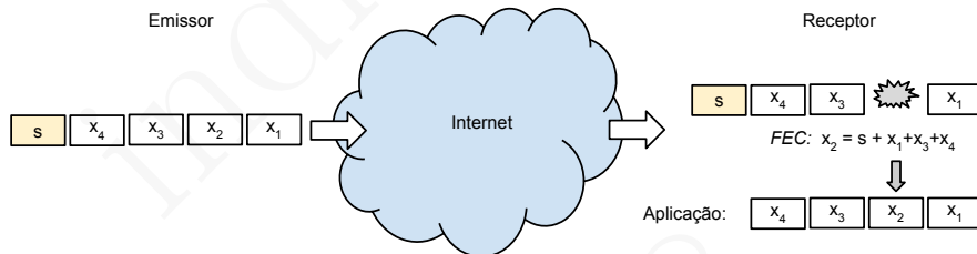
Figura 9.9: Correção de erros de omissão usando Forward Error Correction com base em informação redundante em sumários
