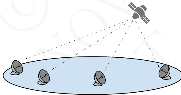
Figura 2.10: Canal de dados baseado em satélite
