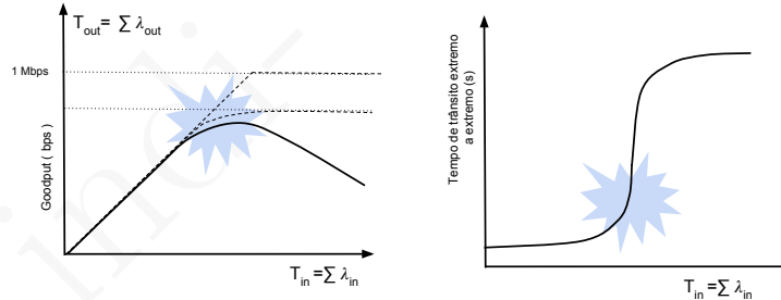
Figura 8.8: Goodput e tempo de trânsito numa rede saturada
