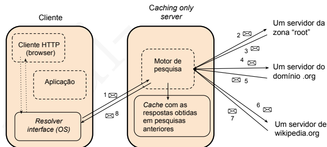
Figura 11.6: Progresso da consulta [name: www.wikipedia.org , type: A ] recursiva enviada a um servidor caching only . O servidor desconhece a resposta e executa uma consulta iterativa.
