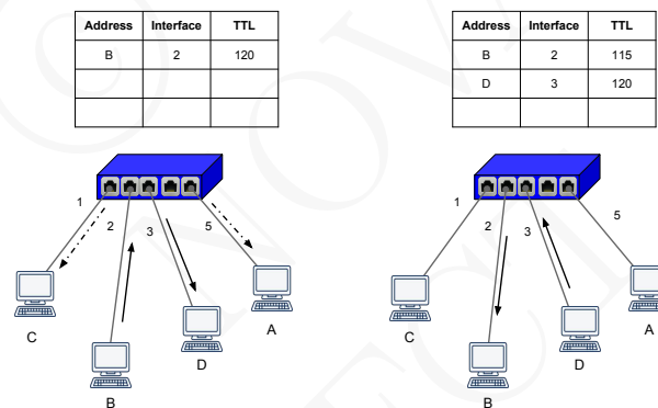
Figura 15.2: Encaminhamento por inundação e aprendizagem pelo caminho inverso: B envia um pacote a D, depois D responde a B. As setas a ponto e traço representam mensagens inúteis.
