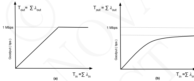
Figura 8.5: Débito útil ( goodput ) com filas de espera infinitas: (a) sem retransmissão de pacotes pelos emissores, (b) com retransmissão prematura de pacotes
