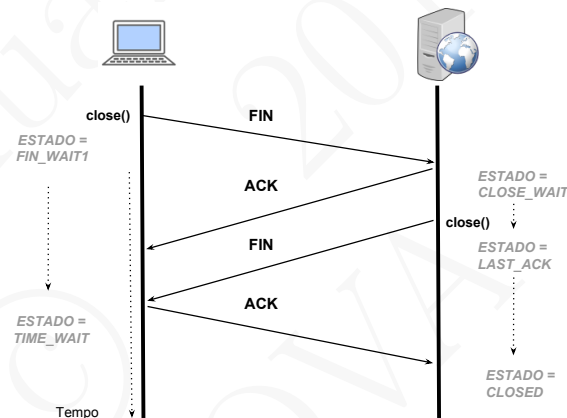
Figura 7.13: Protocolo de fecho de uma conexão TCP
