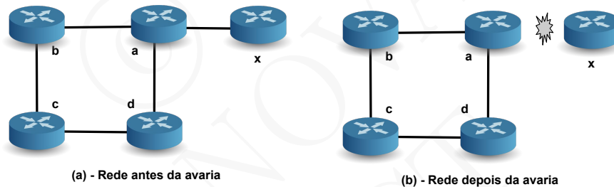
Figura 16.18: Rede onde a solução “ split horizon with poison reverse ” pode não resolver o problema da contagem para o infinito.
