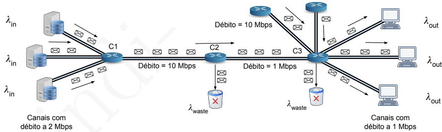
Figura 8.6: Modelo de rede com filas de espera finitas e supressão de pacotes
