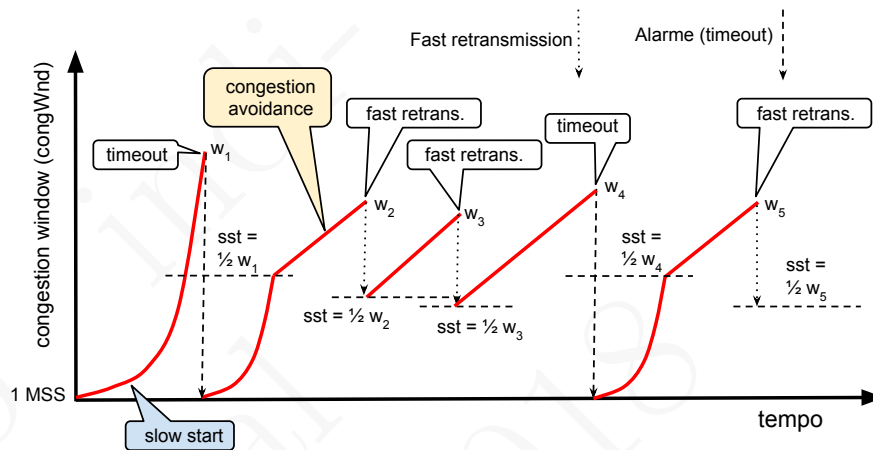
Figura 8.18: Evolução do valor do limite congestion window ao longo de uma conexão TCP na versão TCP Reno (fase fast recovery omitida)
