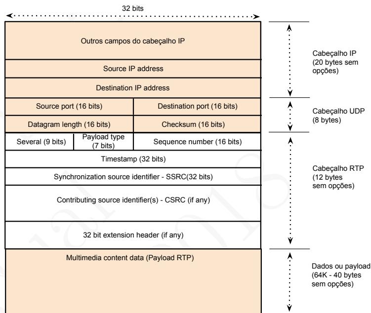
Figura 9.15: Cabeçalho do protocolos RTP
