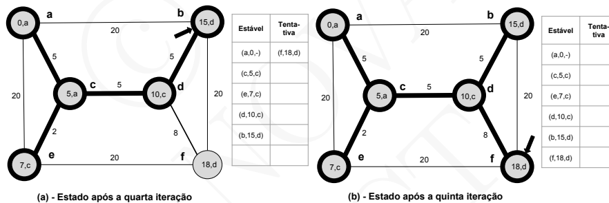
Figura 16.4: Estado do grafo após a quarta iteração (a) e após a quinta e última iteração (b). À direita de cada grafo figura a visão do encaminhamento pelo nó a .
