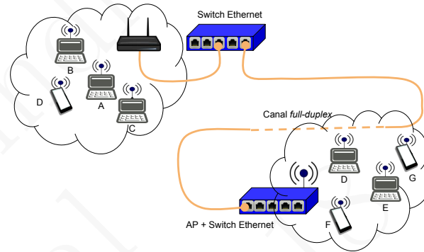
Figura 14.18: Sistema com vários APs interligados por uma rede baseada em switches Ethernet. Os APs funcionam também como switches e um dos switches é simultaneamente também um AP.
