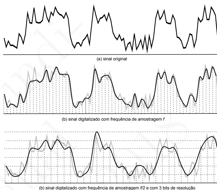
Figura 9.2: Impacto da frequência de amostragem e da resolução no sinal digitalizado
