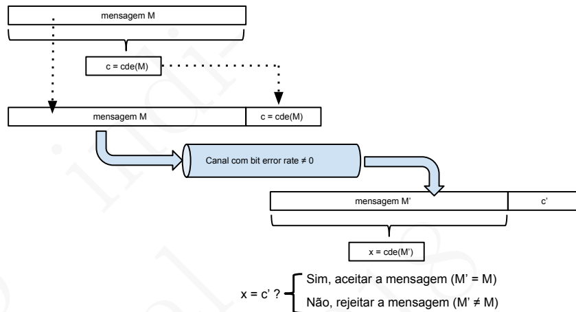
Figura 2.13: Utilização de um código de detecção de erros para controlar se uma mensagem é ou não alterada durante a transmissão pelo canal
