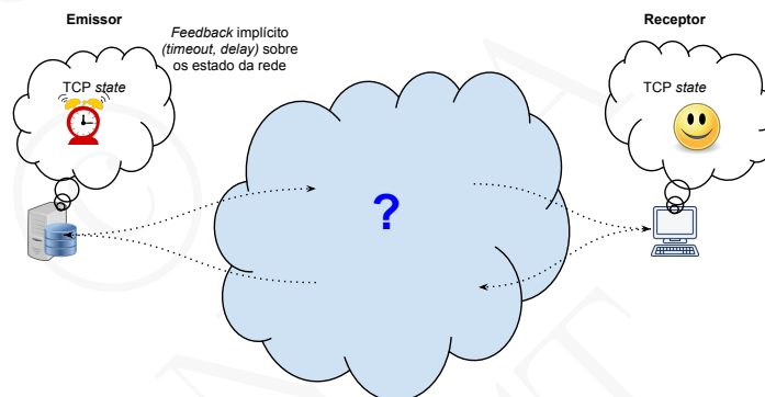
Figura 8.13: Controlo da saturação com base em feedback implícito
