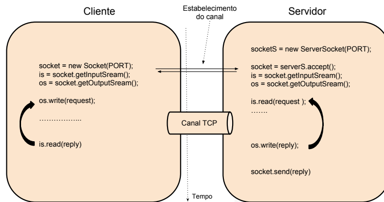
Figura 5.7: Comunicação entre um cliente e um servidor através de um canal TCP
