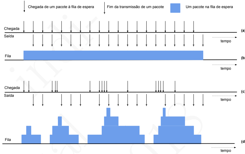
Figura 3.12: Evolução do estado da fila de espera de saída do comutador (Figura 3.11) nas situações: (a) e (b) apenas o computador A emite continuamente pacotes; em (c) e (d) pacotes dos computadores A e B chegam de forma irregular e descoordenada à fila de saída do comutador
