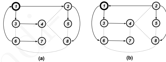
Figura 15.7: Uso da árvore STP para inundação. A raiz da árvore STP é o switch 1. Encaminhamento de um frame emitido pelo switch 6 (a) e pelo switch 2 (b) usando a árvore calculada pelo STP.
