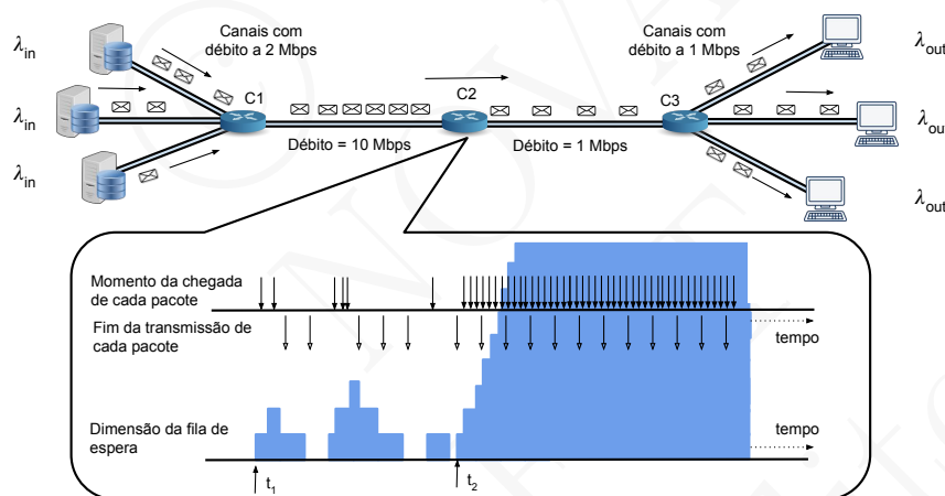
Figura 8.4: Filas de espera no interior da rede com T_{out} = T_{in} de t_1 a t_2 e T_{out} > T_{in} a partir de t_2
