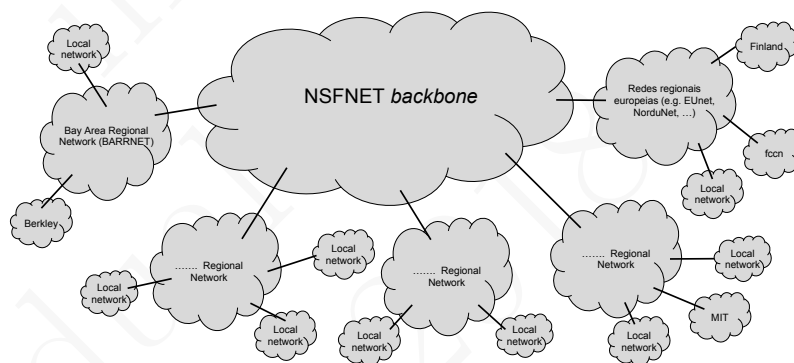
Figura 18.2: Estrutura da Internet pré-comercialização com exemplos de redes regionais e locais
