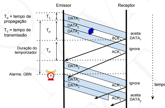
Figura 6.14: Ilustração do mecanismo GBN na sequência do disparo de um alarme
