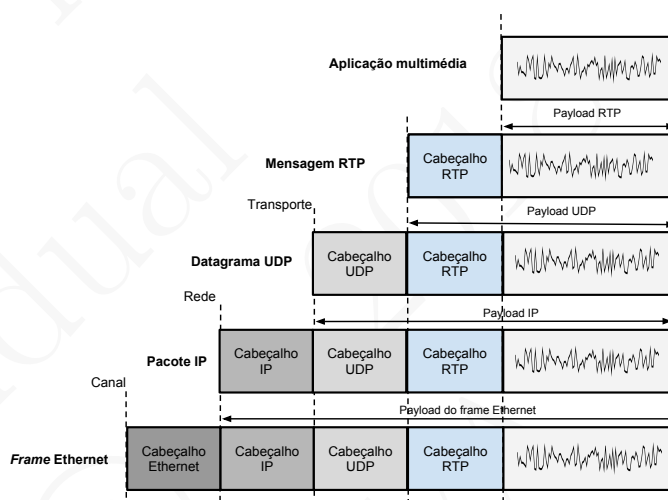
Figura 9.14: Inserção do protocolo RTP na pilha de protocolos TCP/IP
