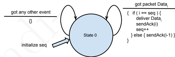
Figura 6.24: Máquina de estados do receptor stop & wait
