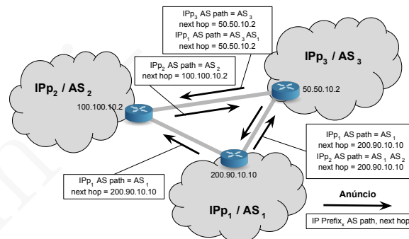
Figura 18.6: Utilização dos anúncios BGP para tomar decisões políticas sobre as escolhas de encaminhamento.
