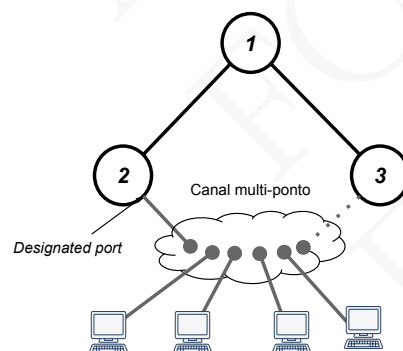
Figura 15.10: Eleição da designated port num canal multi-ponto
