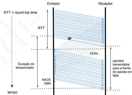
Figura 6.17: Quando a janela é muito grande, o funcionamento GBN leva à potencial retransmissão inútil de muitos pacotes que já foram transmitidos e recebidos para a frente do pacote em falta
