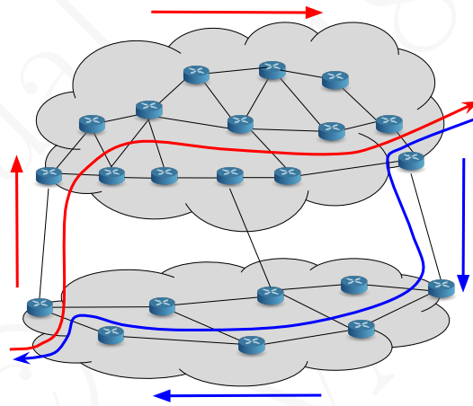
Figura 18.16: Política hot-potato routing e rotas assimétricas.
